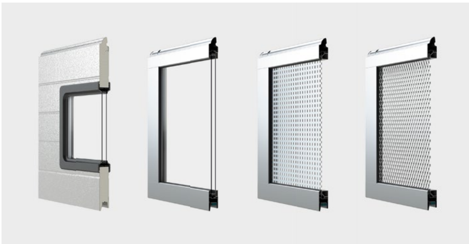
SPESIALSEKSJONER (fra venstre): IS / IA med vinduer, IP med dobbelt glass, IP med perforert plate, IP med aluminium netting/mesh
